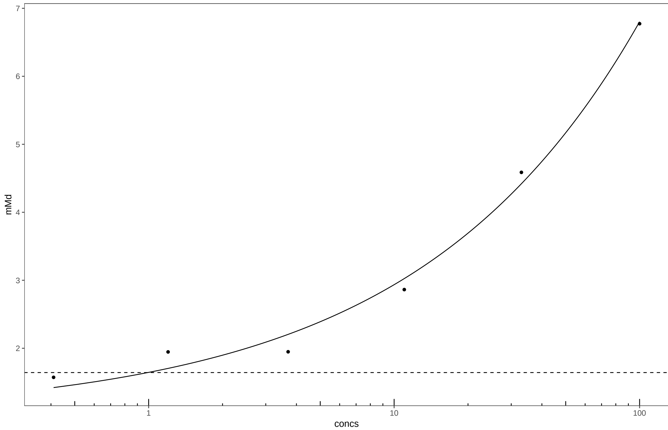
20140903_2-Ethoxy-5-(1-propenyl)phenol_Plate14
