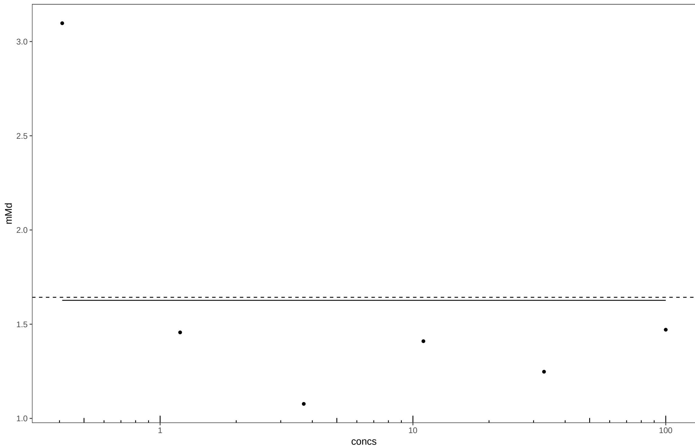
20140903_1-Hexanethiol_Plate13
