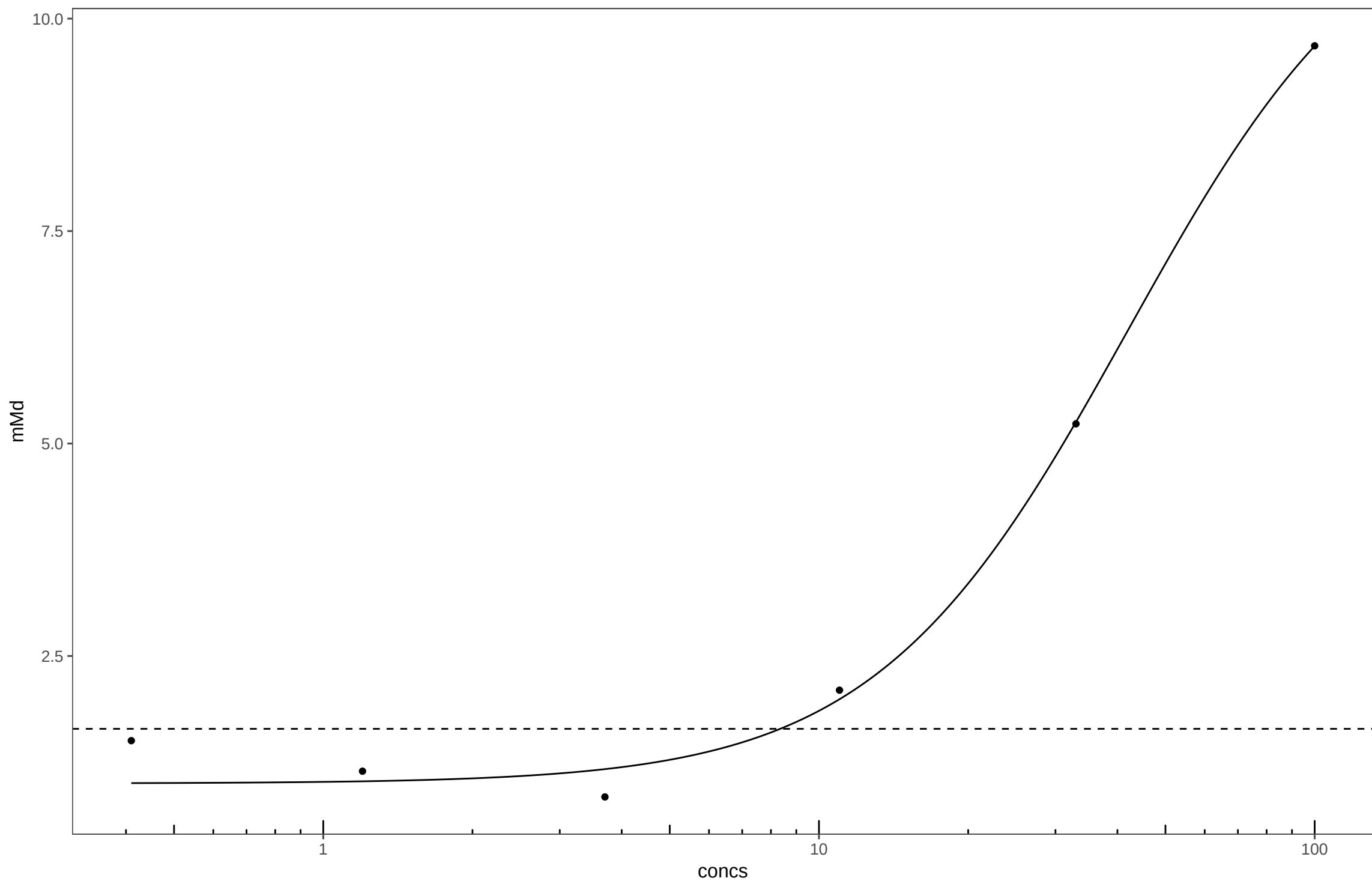
20140402_Fluoranthene_Plate30
