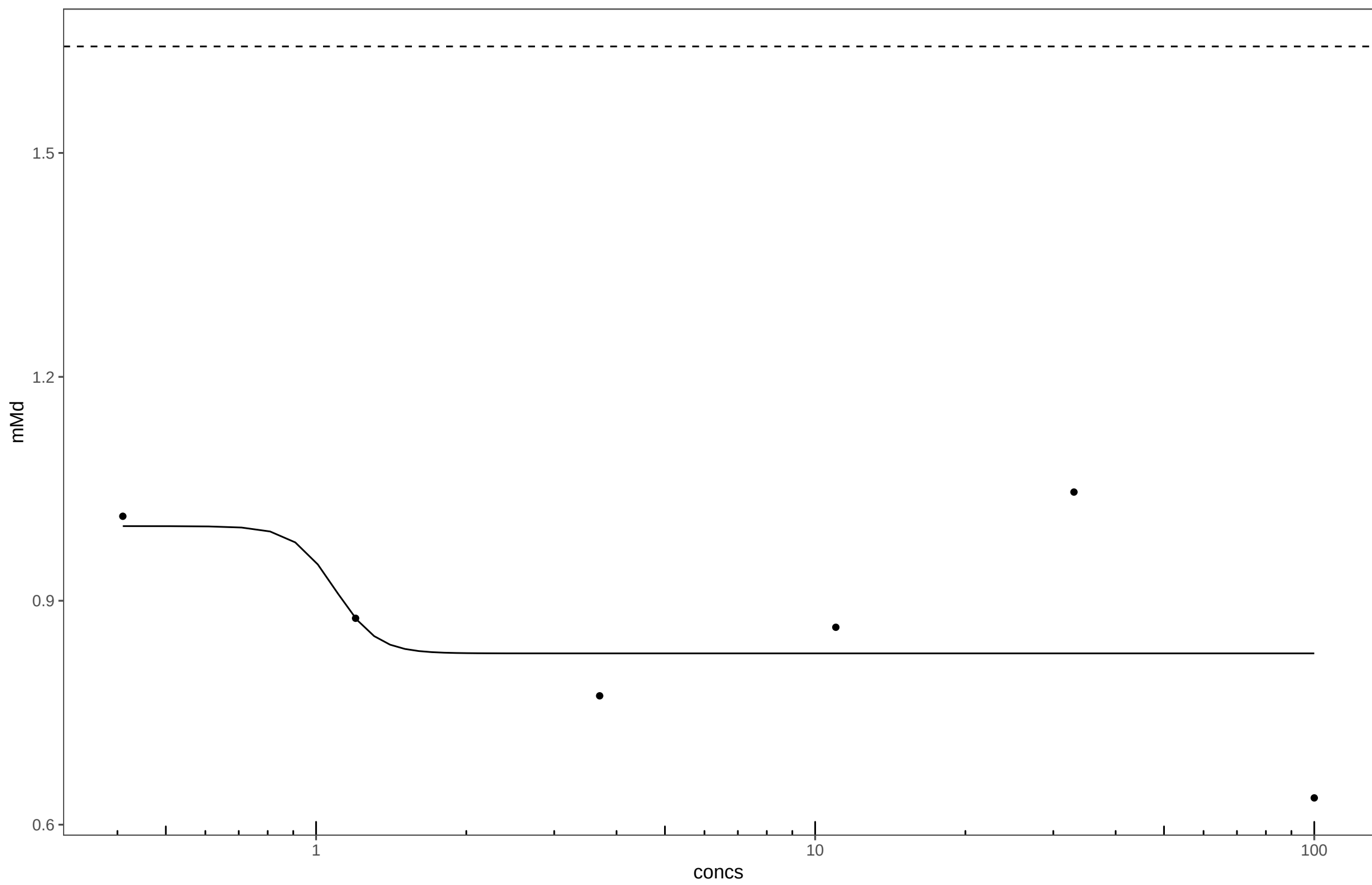
20130321_Daminozide_Plate2
