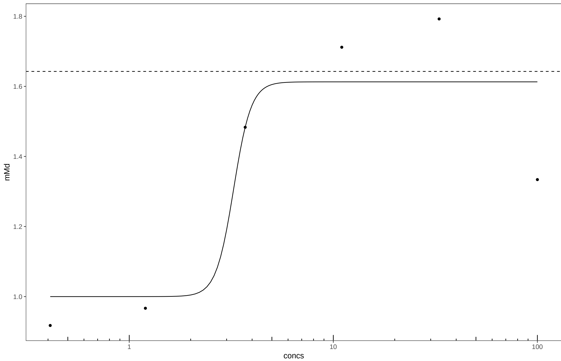
20150610_Damascenone_Plate30
