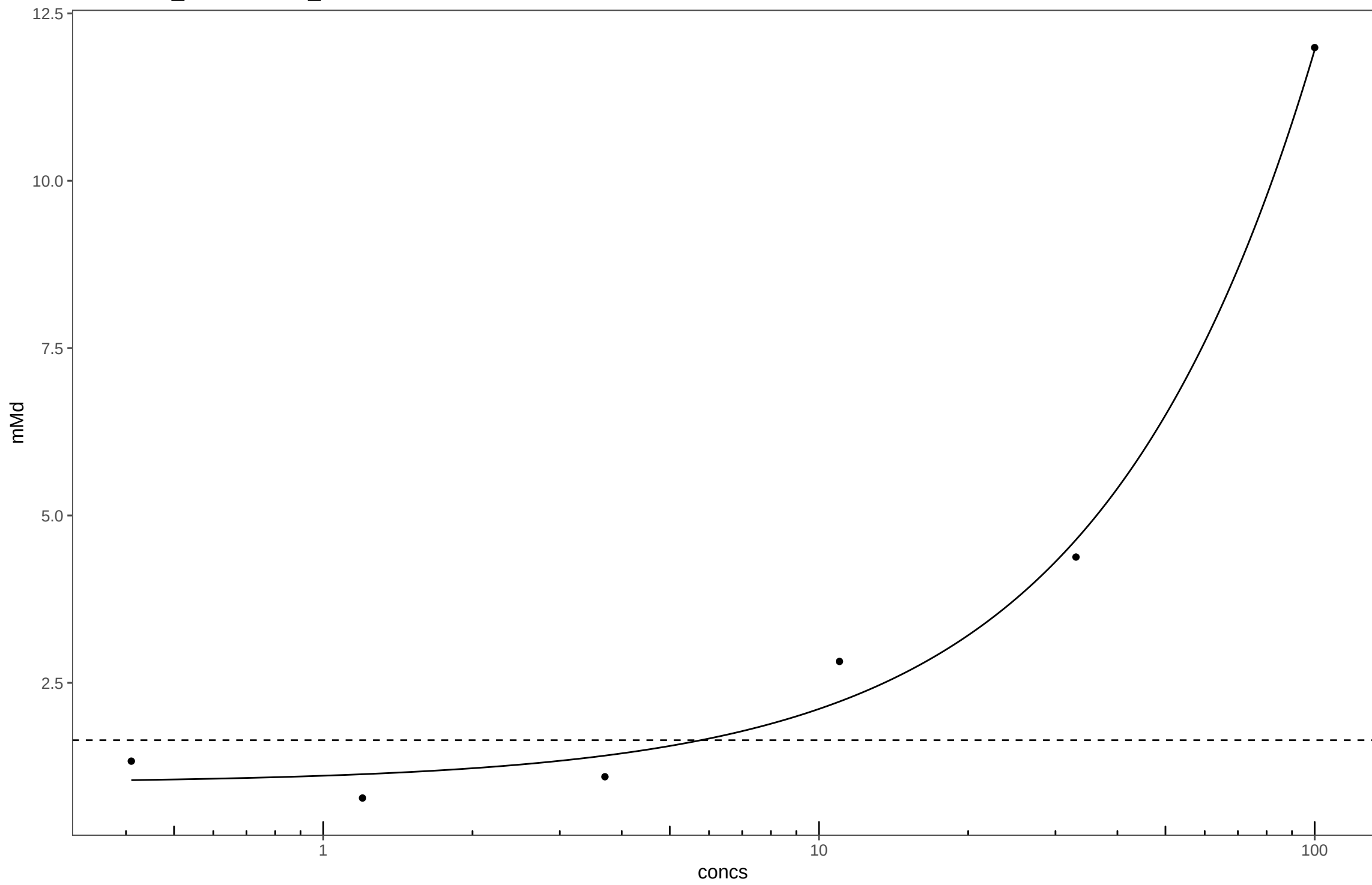
20140409_Endosulfan I_Plate27
