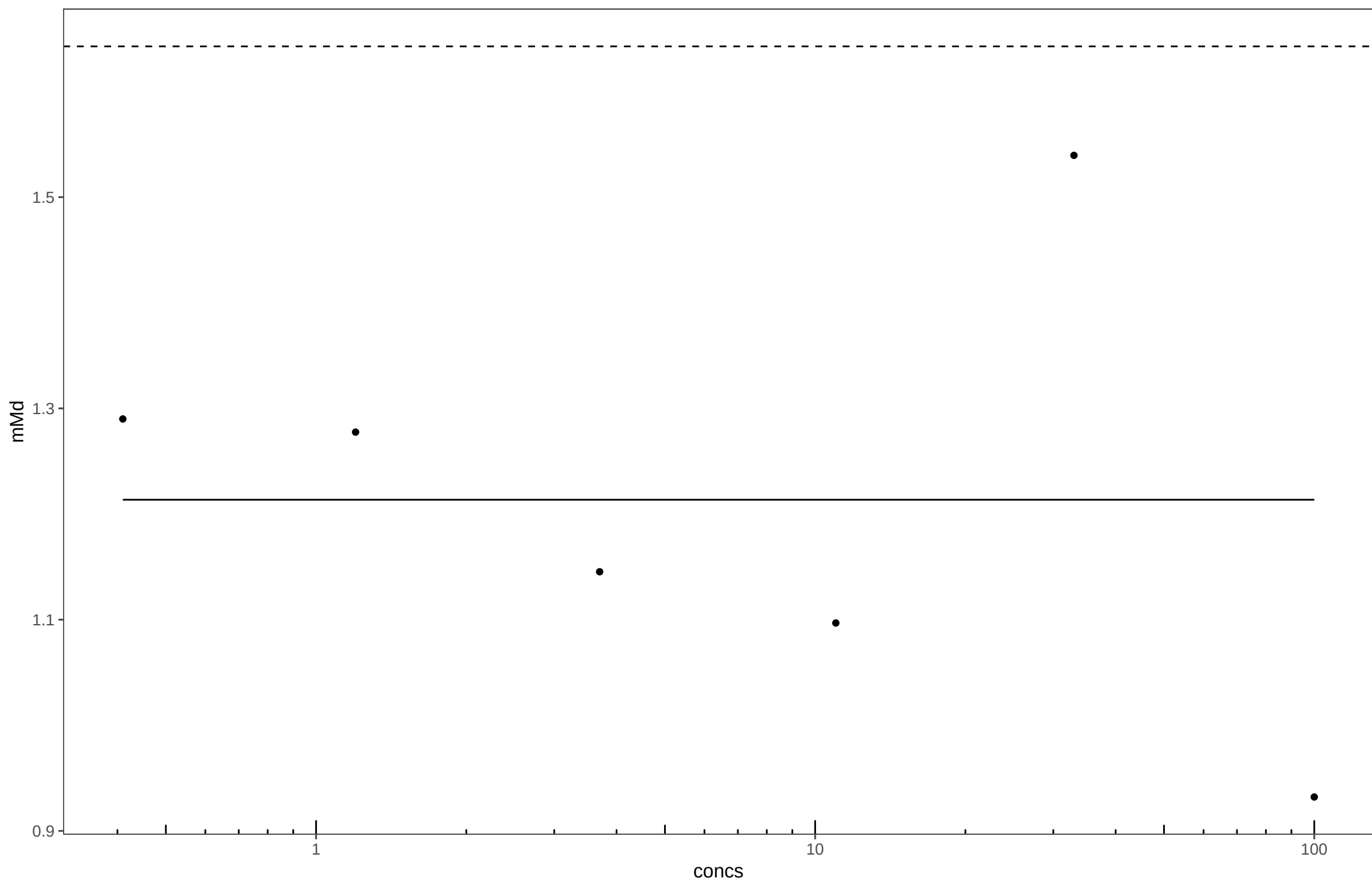
20130321_Imazamox_Plate8
