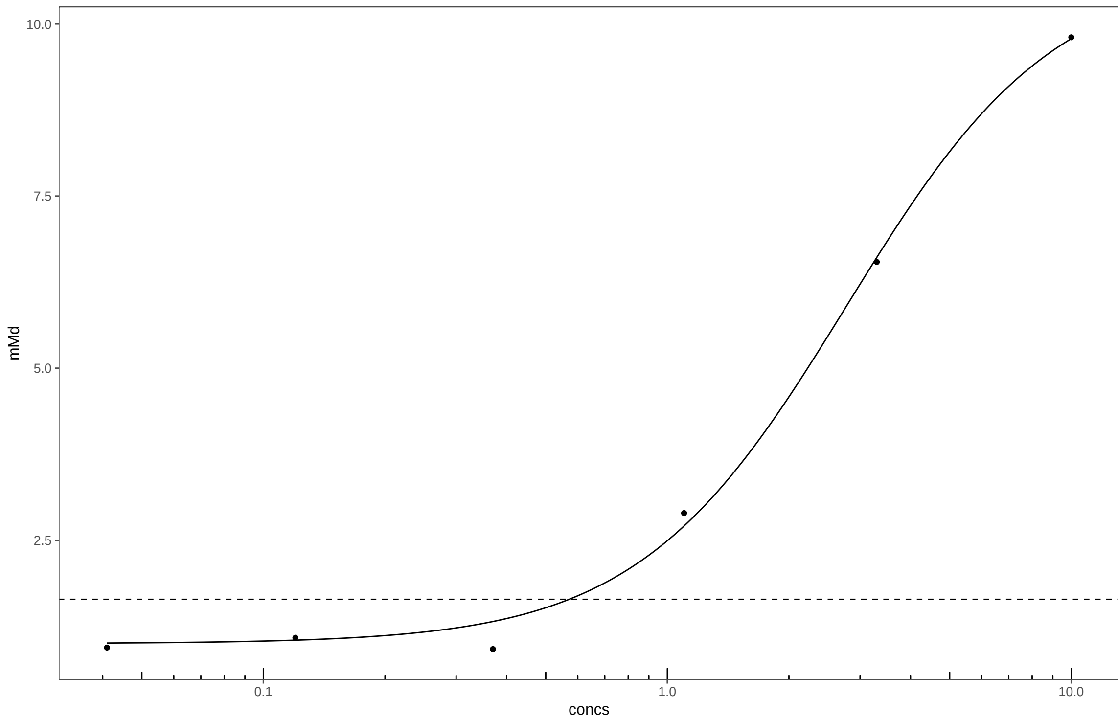
20130321_Oxyfluorfen_Plate2
