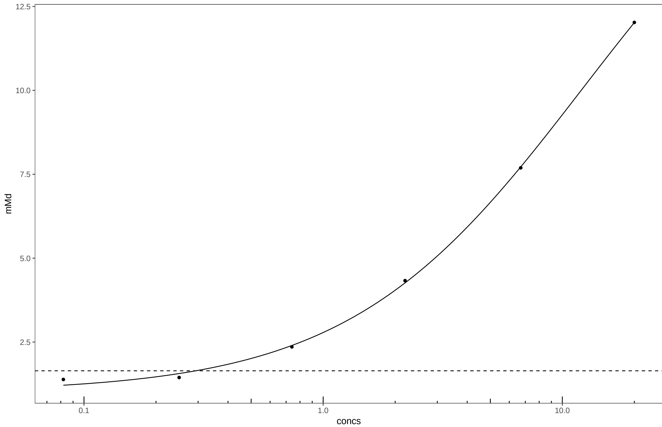
20150610_Lynestrenol_Plate40
