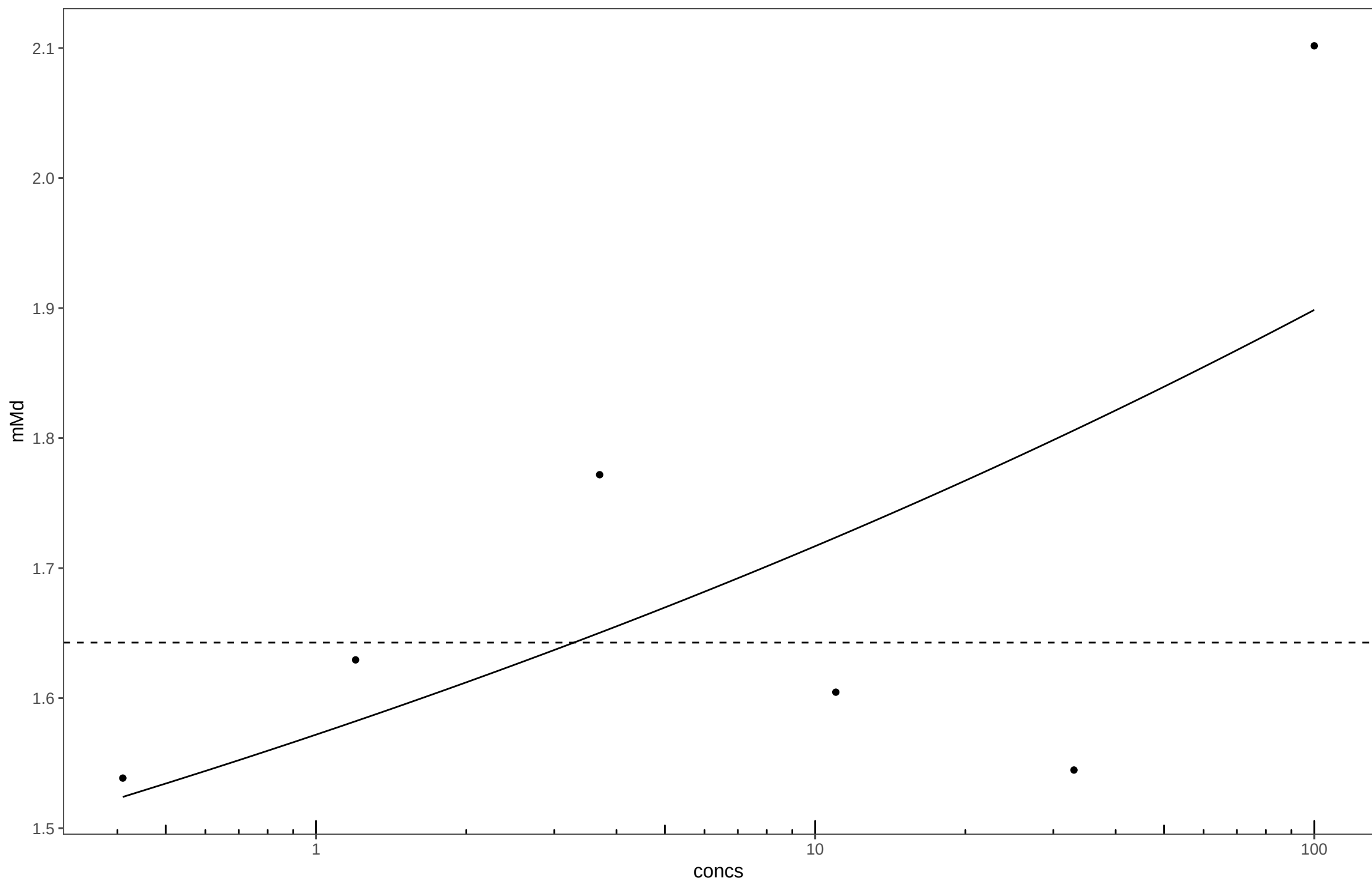
20140326_Metalaxyl_Plate4
