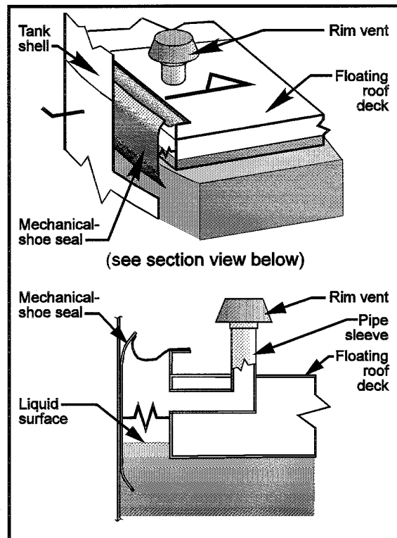
Rim Vent
